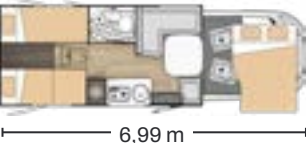
T461 Teilintegriert
