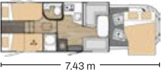
T463 Teilintegriert
