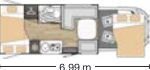
T425 Teilintegriert
