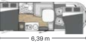
Y881 Teilintegriert
